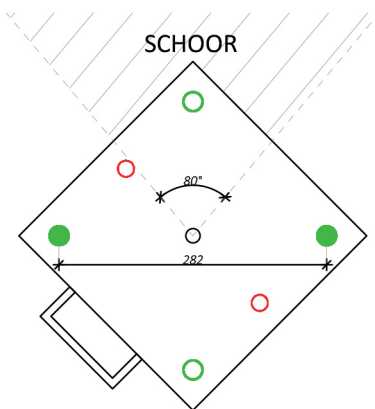
Mafiplaat C met 2 ankers FH II 18 NL SCD diagonaal
