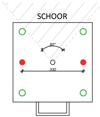
Mafiplaat C met 2 ankers FH II 15 NL SCD optie 2
