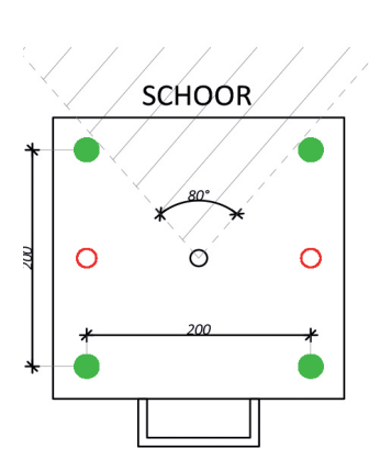
Mafiplaat C met 4 ankers FH II 18 NL SCD
