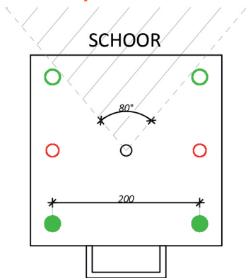
Mafiplaat C met 2 ankers FH II 15 NL SCD optie 1
