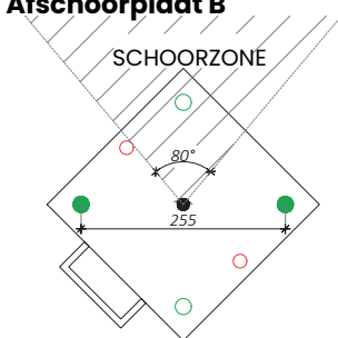
Mafiplaat B met 2 ankers
