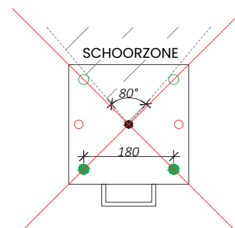
h.o.h. ankers < 200 mm Mafiplaat B met 2 ankers
